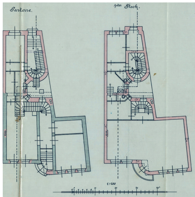
1. att. Ēkas pārbūves 1. un 2. stāva plāni. 1910. gada 17. septembra projekta fragments. Inž. O. F. Hakels.
