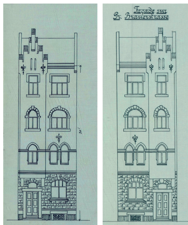
6. att. Aldaru ielas fasādes. No kreisās – 1910. gada 17. septembrī (nerealizēts) un 1910. gada 23. oktobrī (realizētais variants).
