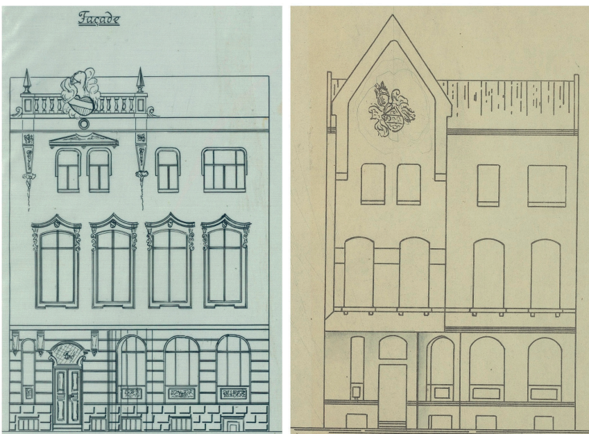
4. att. Atgriežu ielas fasādes. No kreisās – 1910. gada 17. septembrī, 1910. gada 2. decembrī (nerealizētais variants) un 1911. gada 5. augustā.
