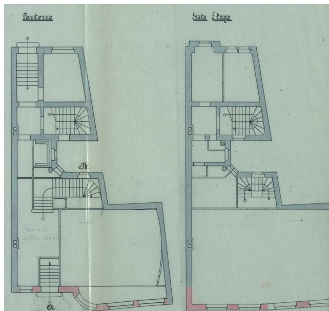
2. att. Ēkas pārbūves 1. un 2. stāva plāni. 1910. gada 2. decembra izmaiņas, projekta fragments. Inž. O. F. Hakels.
