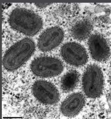
Bakas izraisošais vīruss. Transmisijas elektronmikroskopija, svītra atbilst 200 nm.
