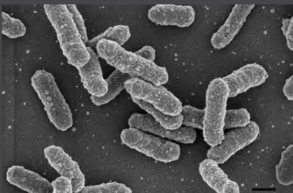
Mēra izraisītāja – Yersinia pestis baktērija. To atklāja Aleksandrs Jersins un Šibasaburo Kitasato Honkongā 1894. gadā. Skenējošā elektronmikroskopija, svītra atbilst 500 nm. Avots: M. Ozel, G. Holland, R. Reissbrodt, www.rki.de
